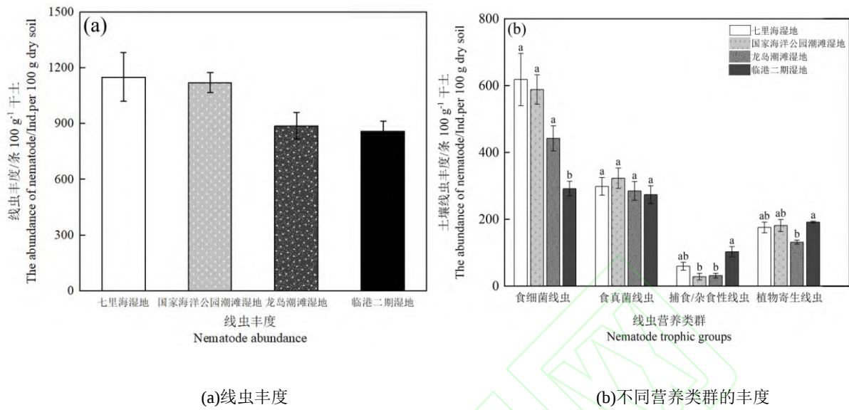
图 1 不同湿地土壤线虫丰度和不同营养类群的丰度
