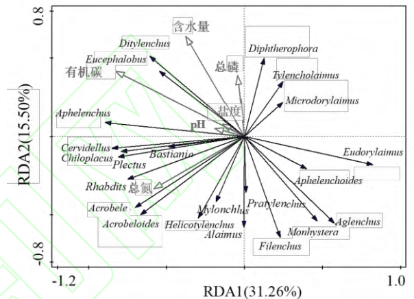
图 3 不同湿地土壤线虫群落 RDA 分析
