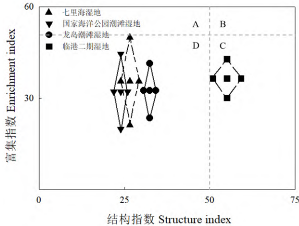
图 2 不同湿地土壤线虫区系分析(基于线虫代谢足迹)
