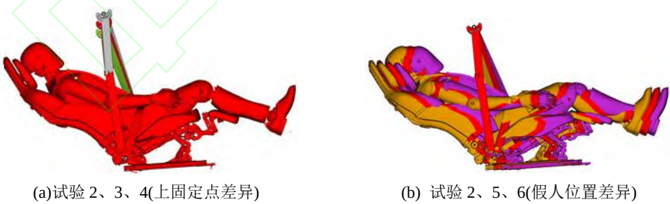
图 6 安全带上固定点设置及假人位置差异
