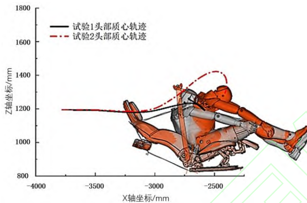
图 2 假人头部运动轨迹对比
