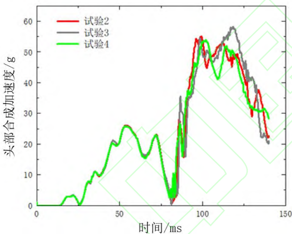
(a) 试验 2、3、4 对比
