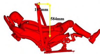
(b) 试验 2 安全带与假人相对位置关系
