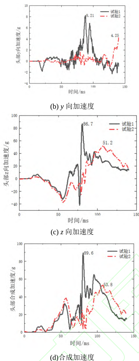
图4 假人头运动学响应
