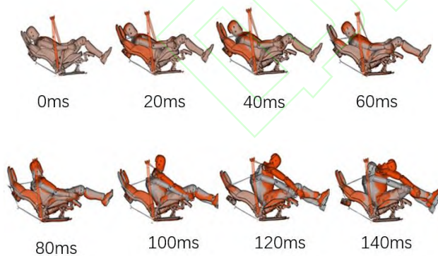
图 3 人体运动学姿态对比
