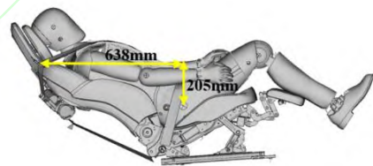
(a) 试验 1 安全带与假人相对位置关系
