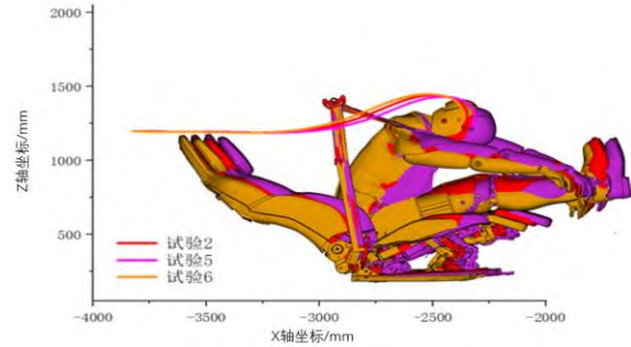
(b) 试验 2、5、6(假人位置差异)
