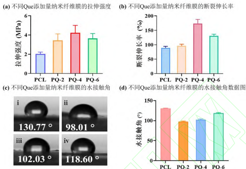
(a) 拉伸强度; (b) 断裂伸长率; (c) 水接触角形貌; (d) 水接触角
