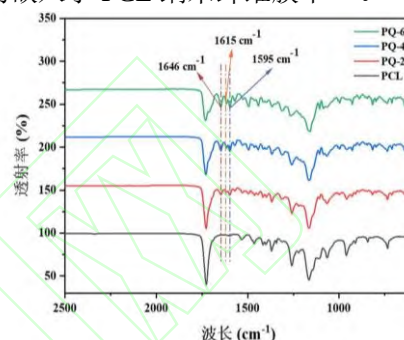
图 2 不同 Que 添加量纳米纤维膜傅里叶变换红外光谱图
