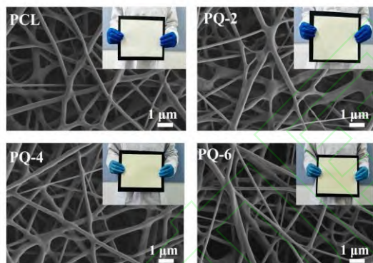
图 1 不同 Que 添加量纳米纤维膜扫描电子显微镜图
