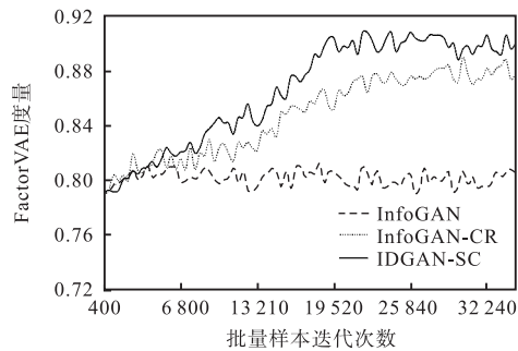
图3 训练过程中不同方法的性能趋势
