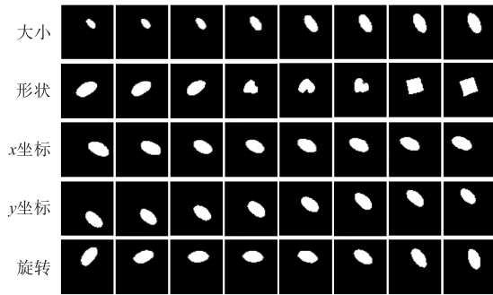
图 4 IDGAN-SC在 dSprites数据集上解耦效果
