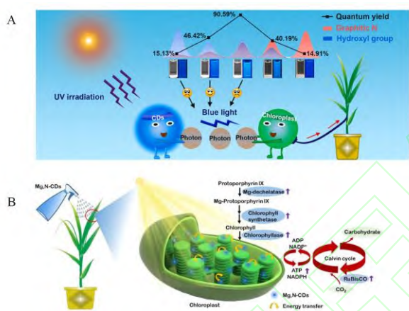
图3 (A)不同荧光量子产率的CDs对光合作用的影响 [47] (B)镁掺杂CDs对水稻叶绿素含量的影响 [34]
