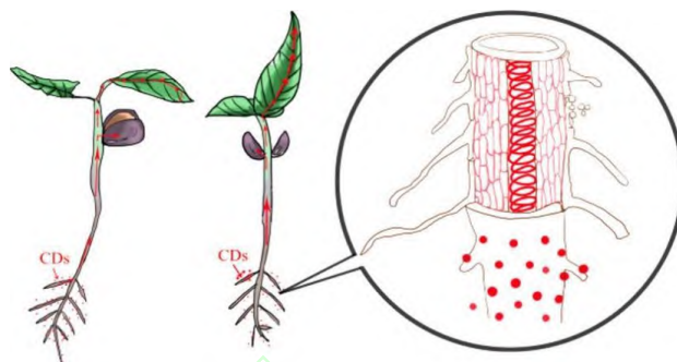
图 2 植物通过根部途径吸收 CDs [44]
