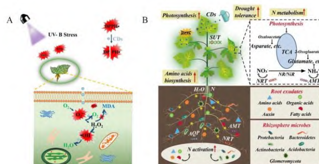
图 4 (A) CDs 清除生菜中 UV-B 胁迫产生的活性氧 [46]
