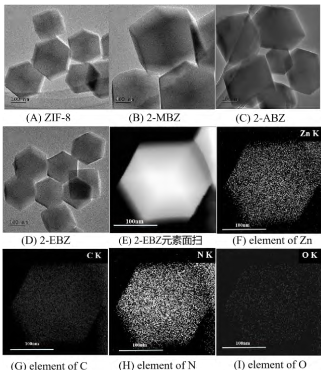
图 3 不同样品的 TEM 图像及 2-EBZ 的元素面扫图像
