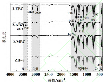
图 4 不同样品的红外光谱图
