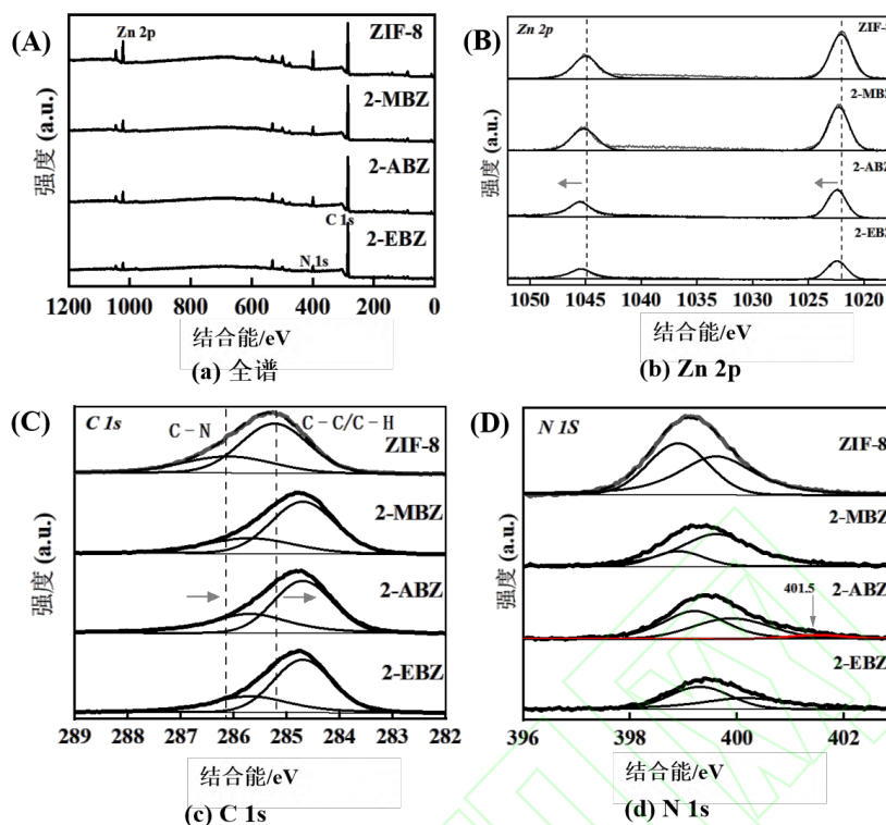
图 5 不同样品的 XPS 谱图
