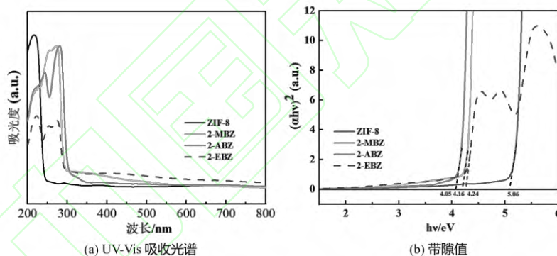
图 6 不同样品的 UV-Vis DRS 谱图及禁带宽度
