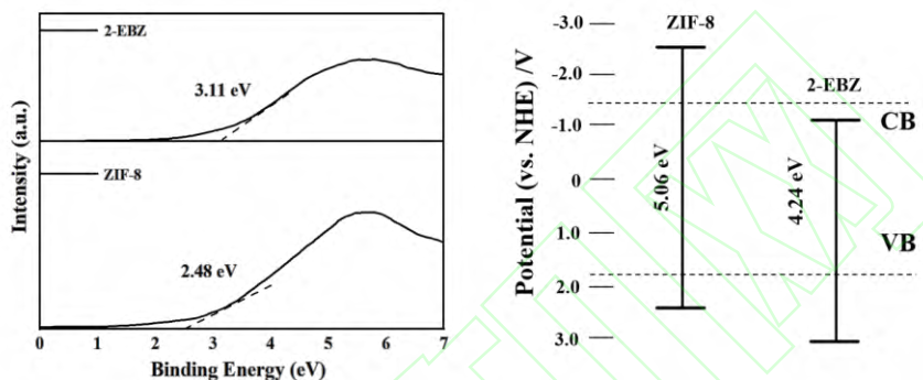
图 8 ZIF-8 与 2-EBZ 的价带谱和能带结构
