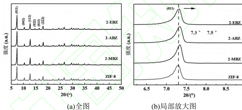
图 2 不同样品的 XRD 图谱
