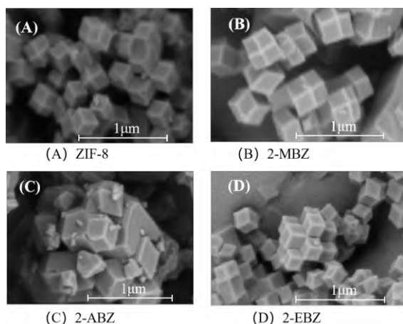
图 1 不同样品的 SEM 图像
