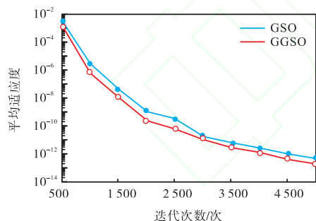
图 4 测试函数 f_{11} 结果对比
