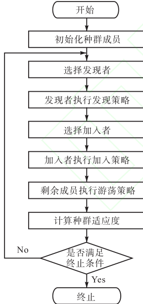
图 1 标准 GSO 算法流程图
