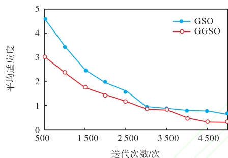
图 3 测试函数 f_6 结果对比
